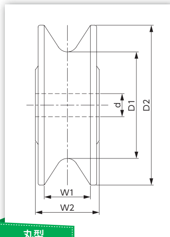
丸型
