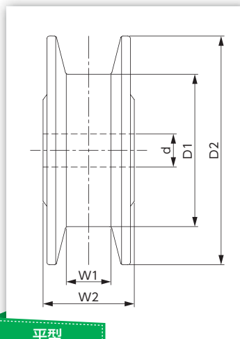
平型
